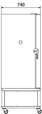
Zijkant
